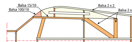
COUPE AXIALE F DE LA CARINE
