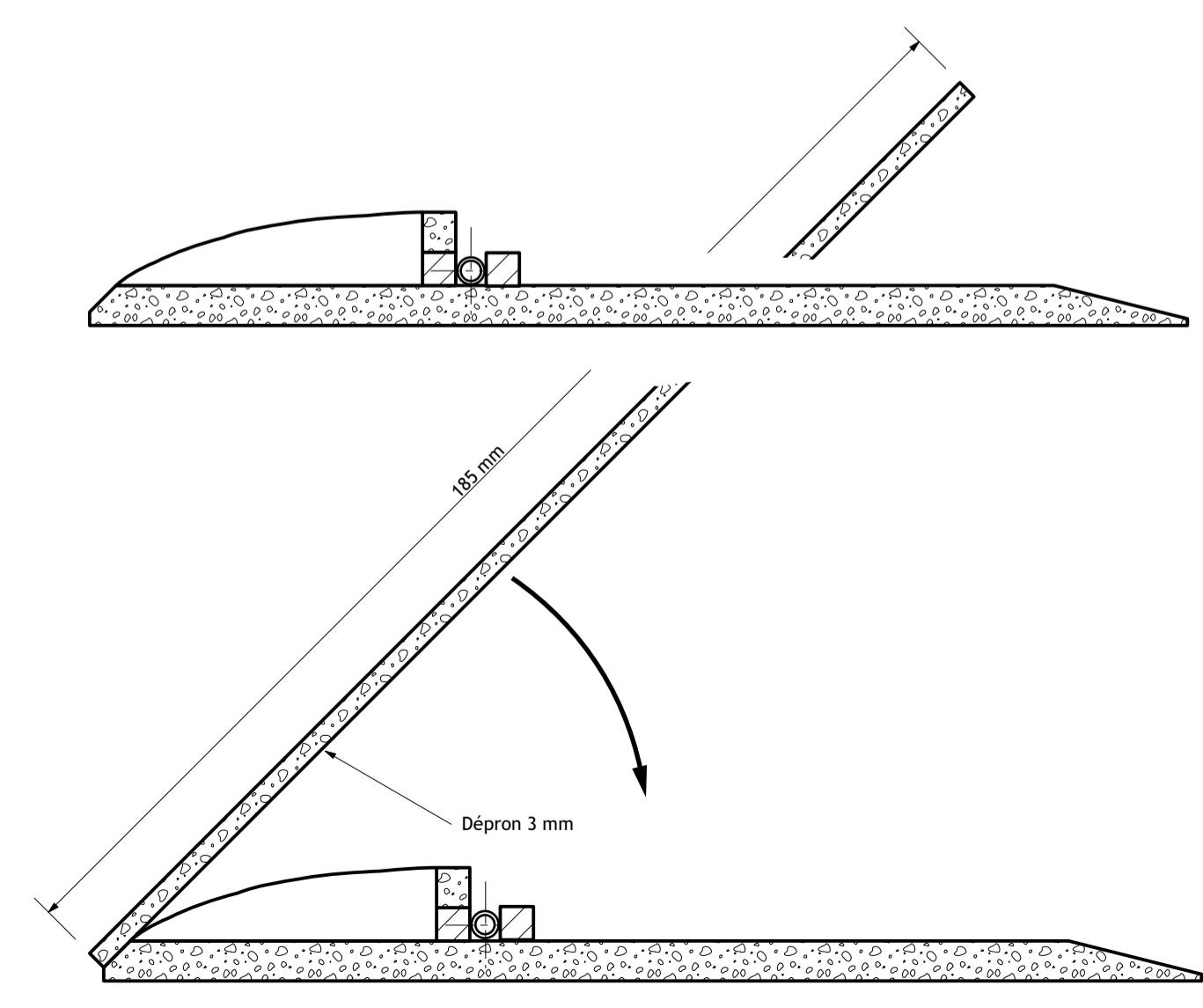
Construction de l'aile (selon coupe A - A)
